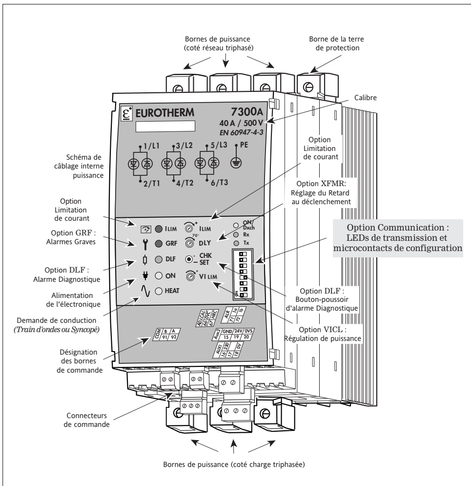
Figure 1-1 Vue générale du gradateur de puissance 7300A calibre de 16 A à 40 A
