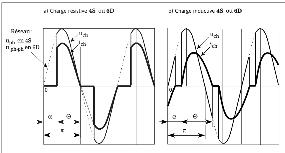
Figure 3-5 Tension et courant d'une phase de charge triphasée (code 4S ou 6D) en «Angle de phase» a) - charge résistive b) - charge inductive.
