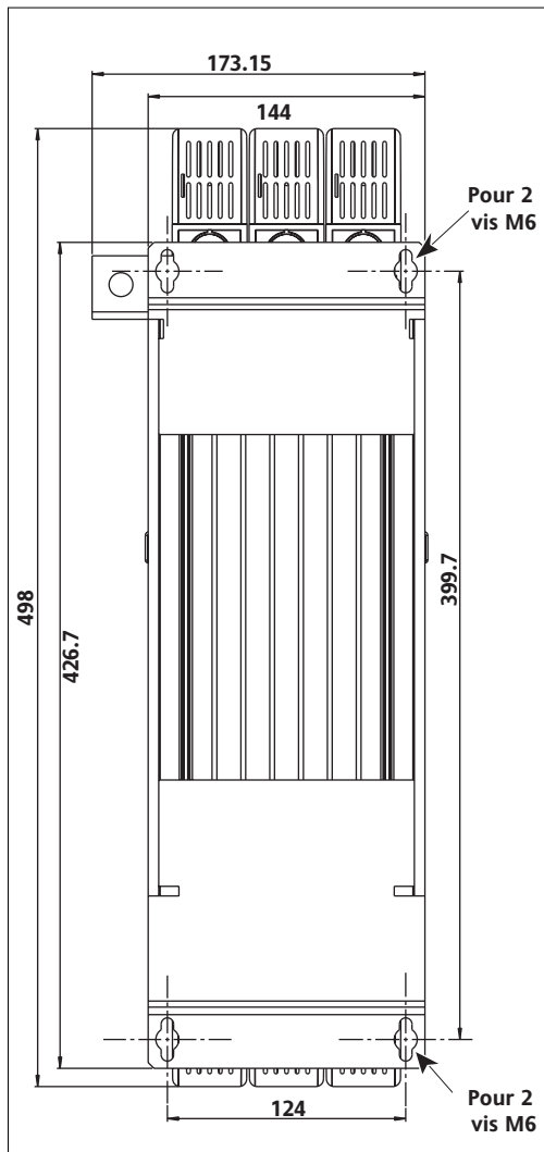
Figure 2-4 Fixation des unités \geq 125 A
