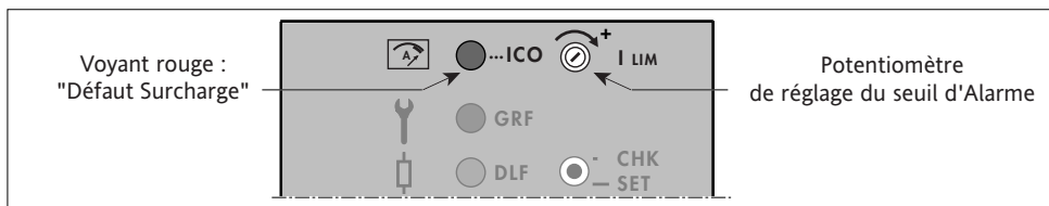
Figure 5-3 Disposition du voyant «ICO» et du potentiomètre «I lim» en Option ICO
