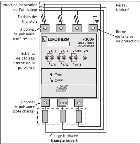
Figure 2-10 Branchement de charge triphasée en Triangle Ouvert (6D)
