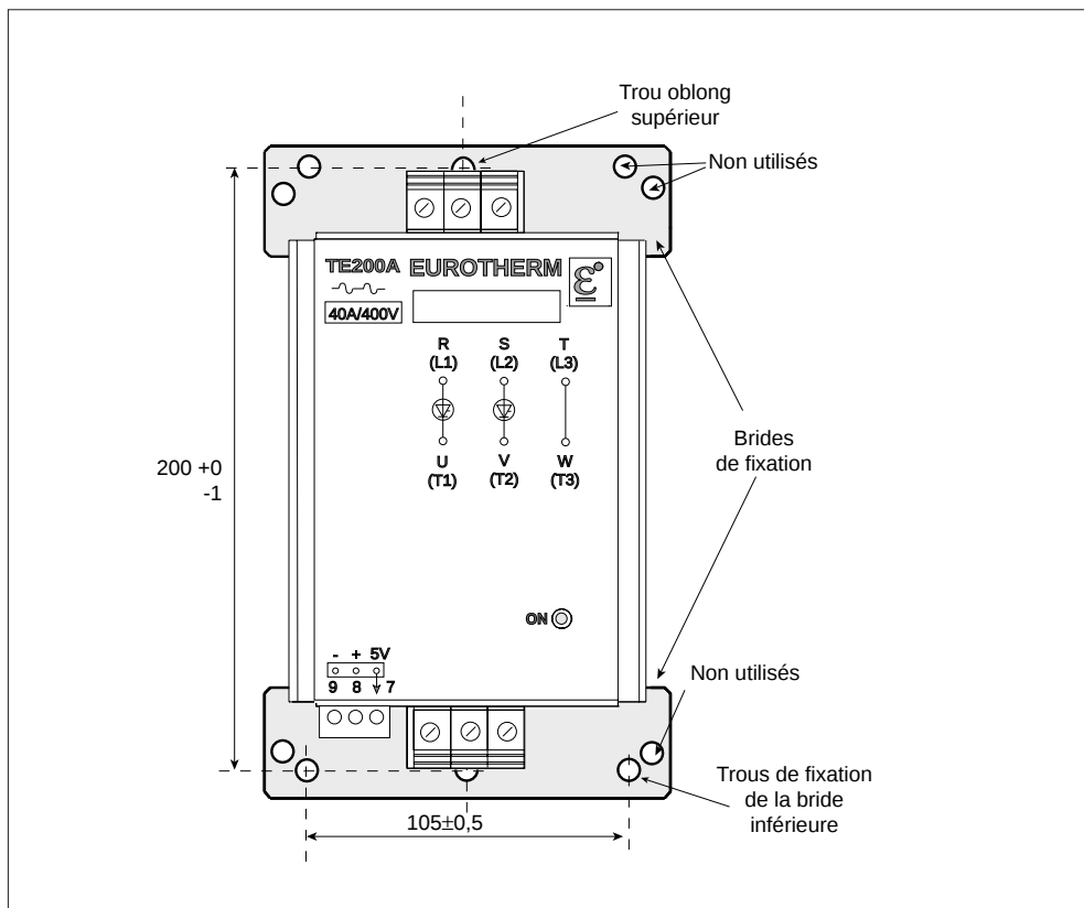
Figure 2-4 Cotes de perçage (en mm) et fixation du gradateur TE200A en fond d'armoire
