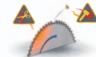
Lame de scie circulaire à denture rapportée (dent projetée)
